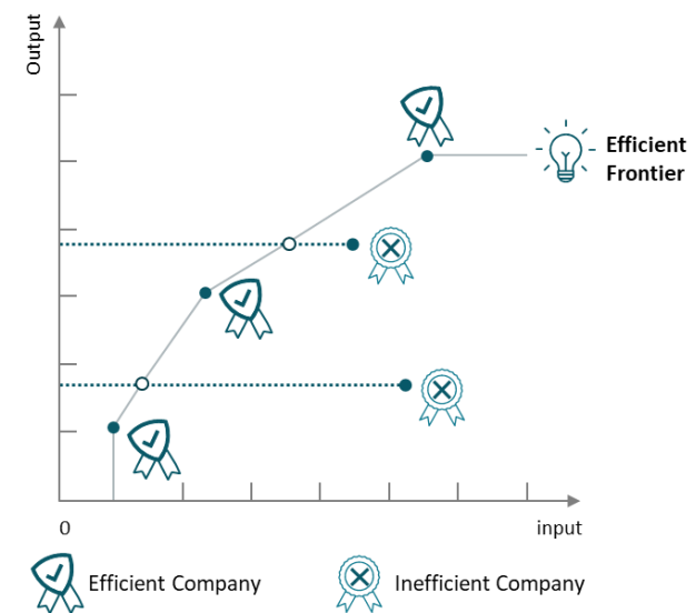
Abb. 1: Efficient Frontier
